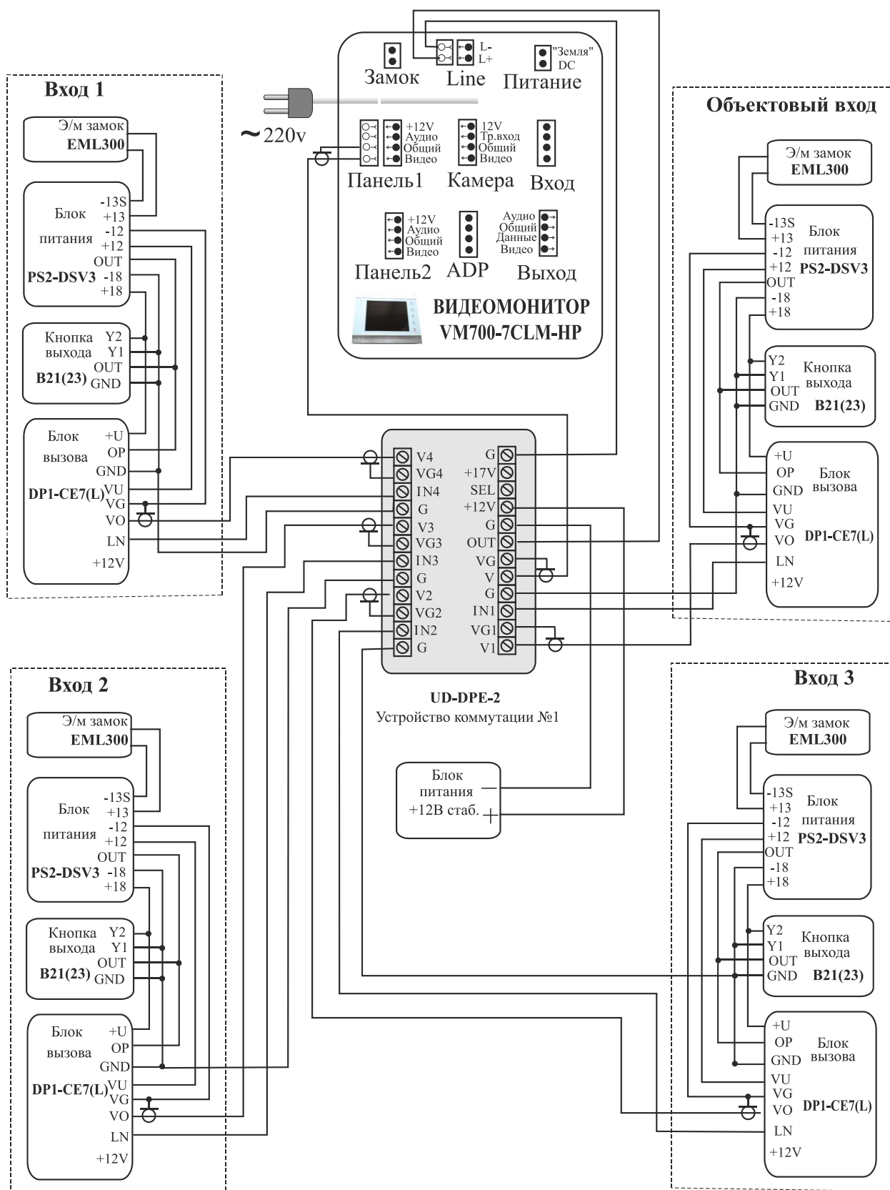
Рис.5 Схема подключения ДК, представленного на рис.3, для VM700
