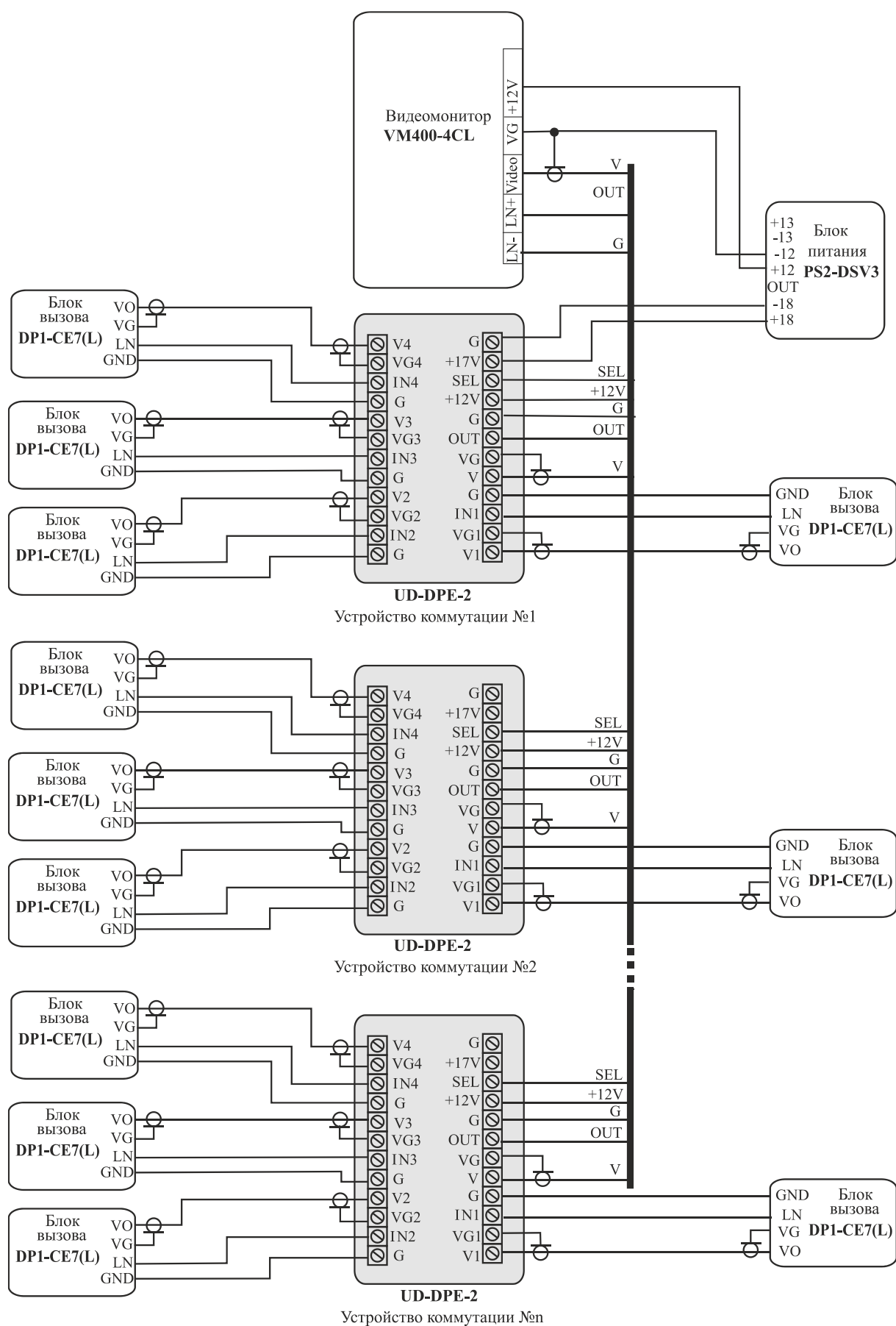
Рис.6 Схема каскадного соединения УК для VM400-4CL
