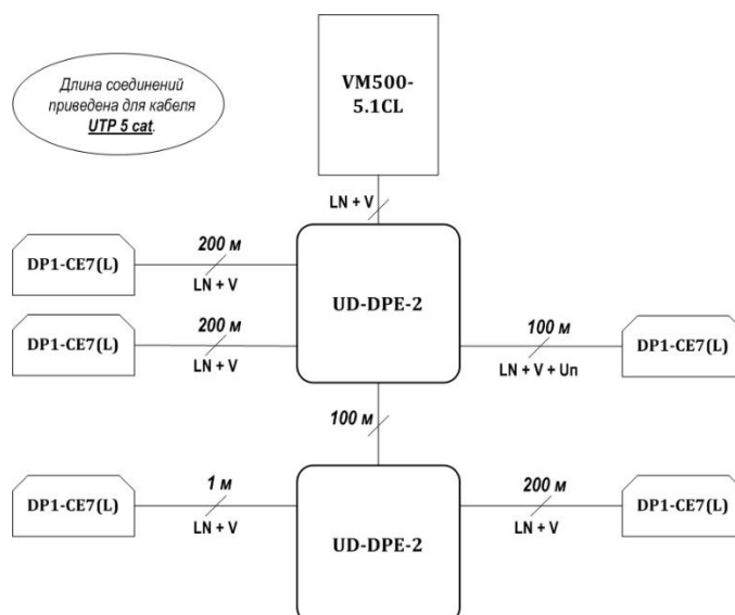
Рис.11 Пример длин кабеля
