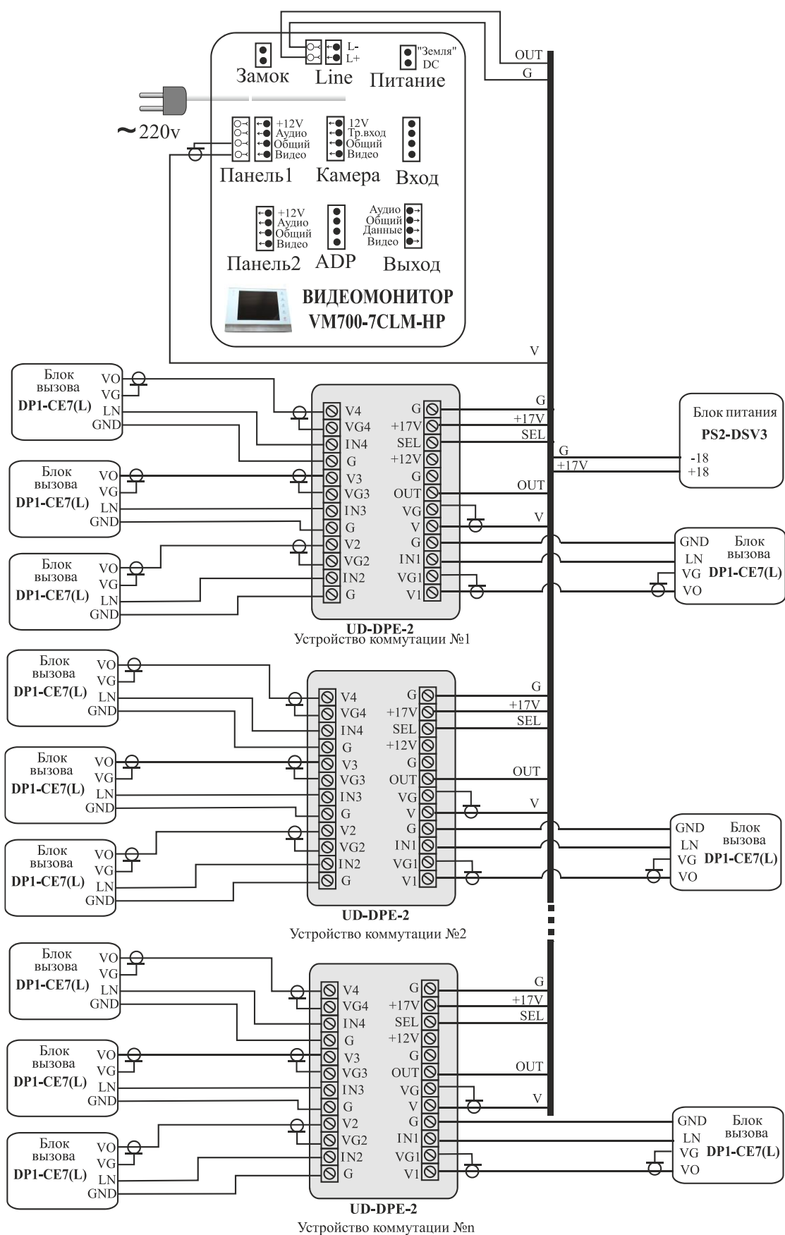
Рис.8 Схема каскадного соединения УК для VM700-7CLM-HP
