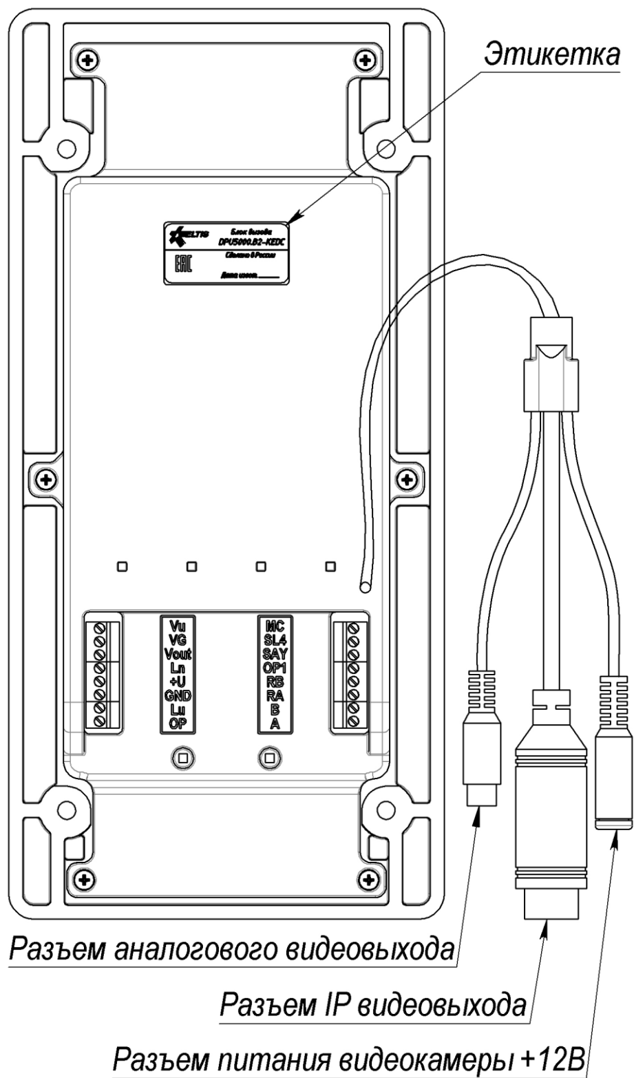
Рис.5 Внешний вид DPU5000-KEDC-T/IP-CVBS со стороны задней крышки
