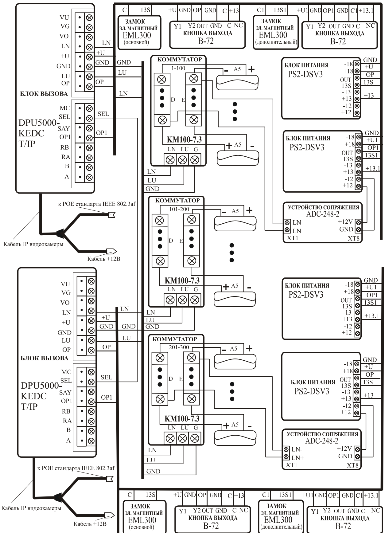
Рис.7 Пример схемы подключения DPU5000 –KEDC-IP в автономном режиме в составе домофонного комплекса (аналог ELTIS303).
