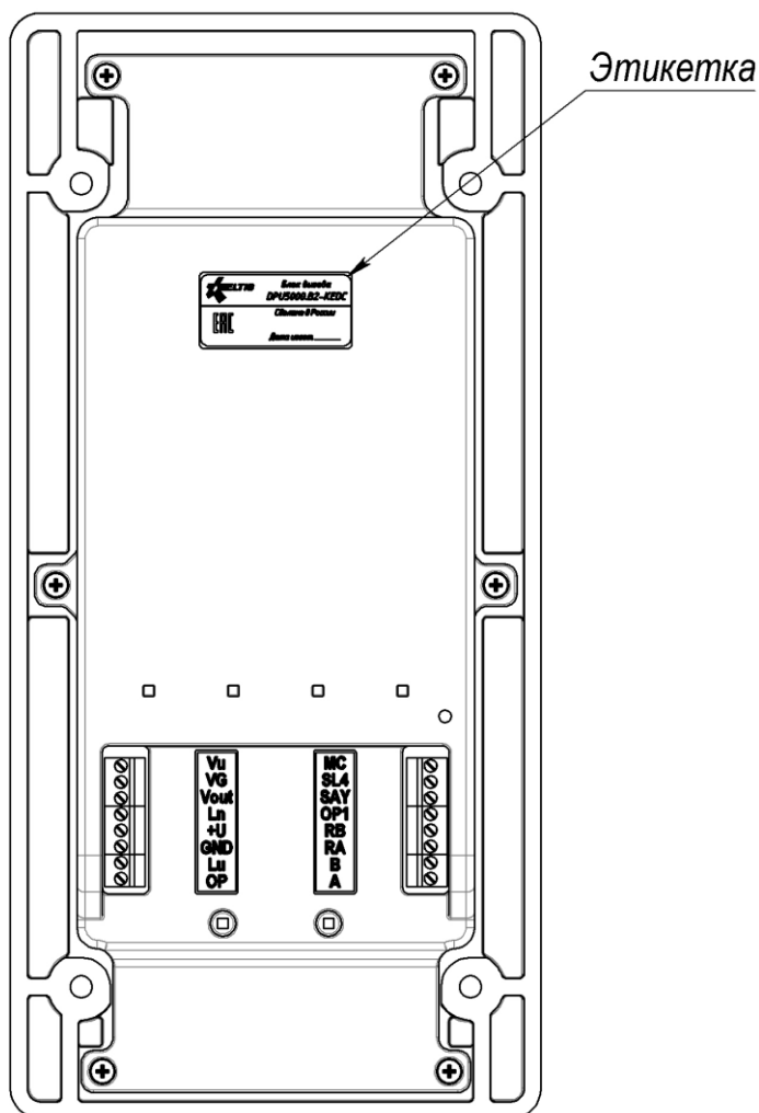
Рис.3 Внешний вид DPU5000-KEDC со стороны задней крышки Описание присоединительных контактов блока вызова:
