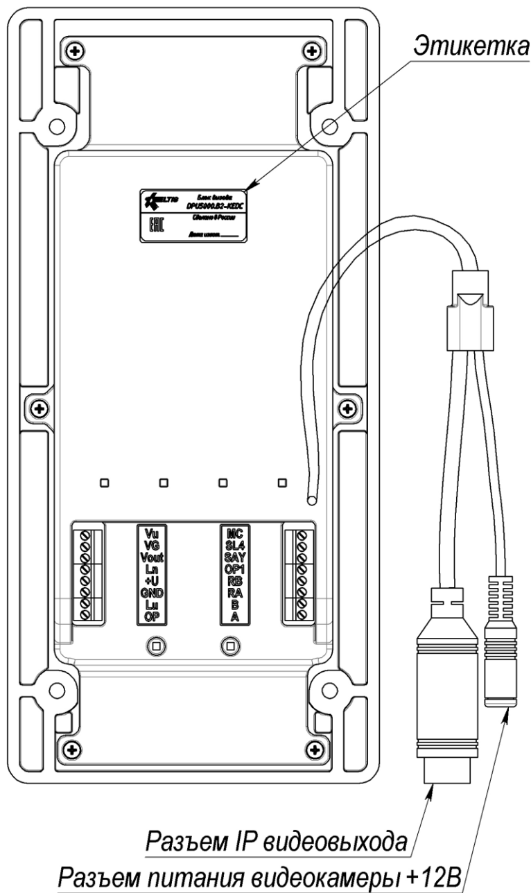
Рис.4 Внешний вид DPU5000-KED-IP со стороны задней крышки
