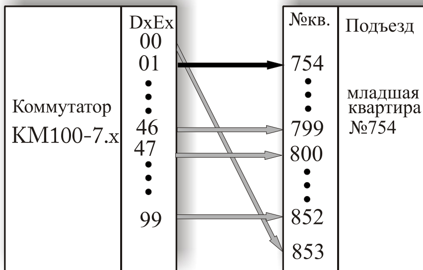
Рис.10а Соответствие выходов коммутатора номерам квартир по умолчанию при np = 1 и номере младшей квартиры равному 754
