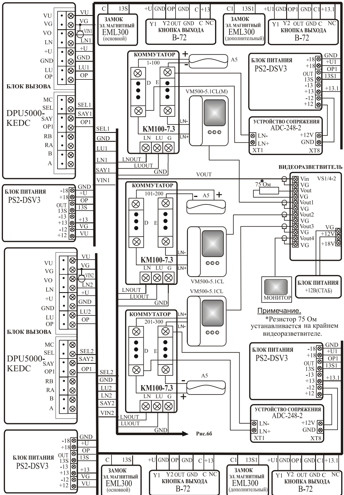
Рис.6а Пример схемы подключения DPU5000-KEDC в автономном режиме в составе домофонного комплекса (аналог ELTIS303).
