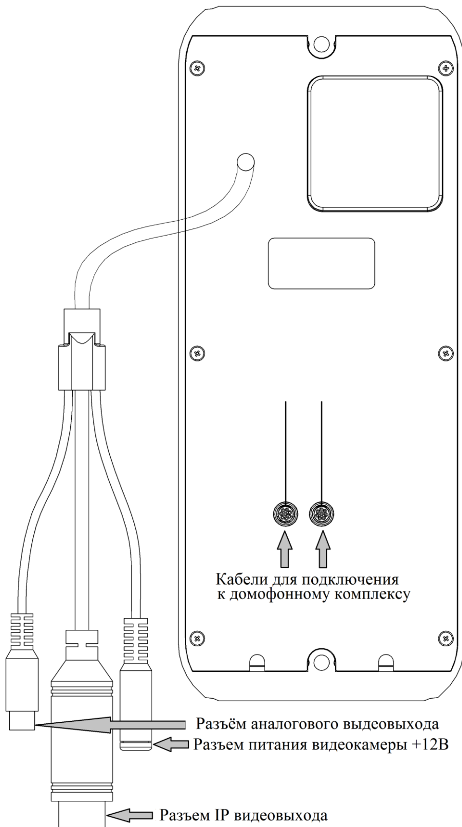
Рис.5 Внешний вид БВ DP5000.B2-KEDC43 T/IP-CVBS и DP5000.B2-KEDC44T/IP-CVBS со стороны задней крышки
