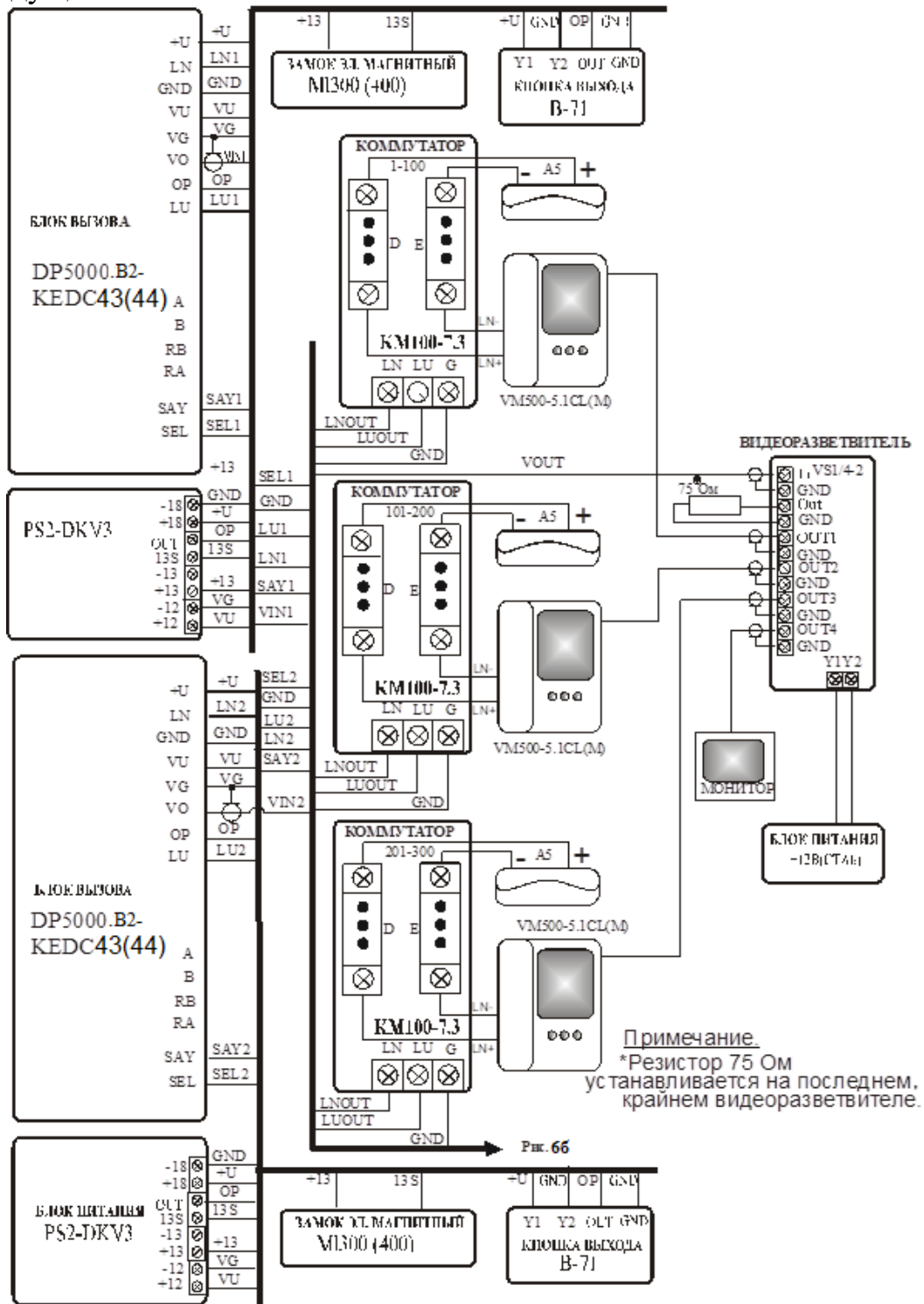
Рис.6а Пример схемы подключения DP5000.B2-KEDC43(44) в автономном режиме в составе домофонного комплекса (аналог ELTIS303).
