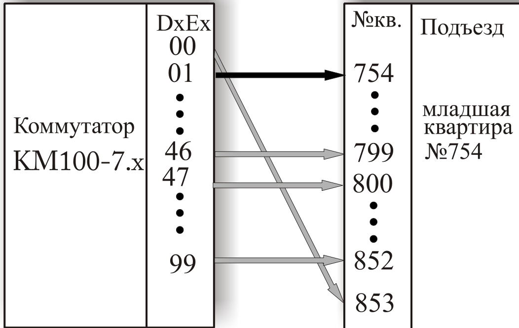
Рис.10а Соответствие выходов коммутатора номерам квартир по умолчанию при pn = 1 и номере младшей квартиры равному 754
