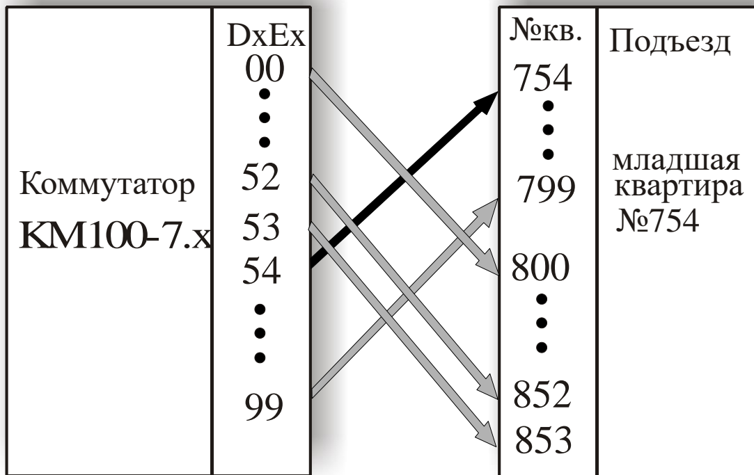
Рис.10б Соответствие выходов коммутатора номерам квартир при установке pn = 54 и номере младшей квартиры равному 754
