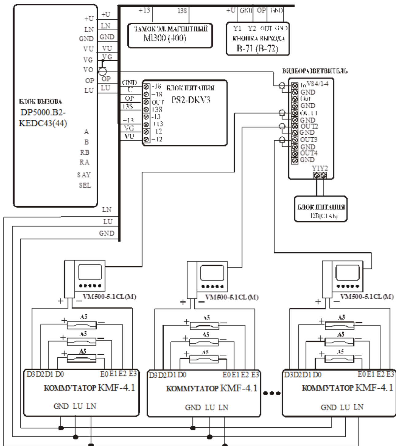
Рис.9 Пример схемы подключения DP5000.B2-KEDC43(44) в автономном режиме в составе домофонного комплекса с этажными коммутаторами
