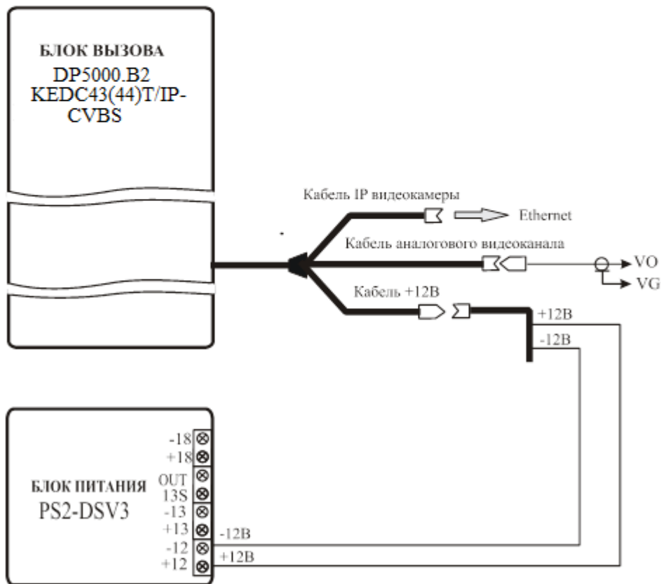
Схема подключения видеотракта к блоку питания +12В
