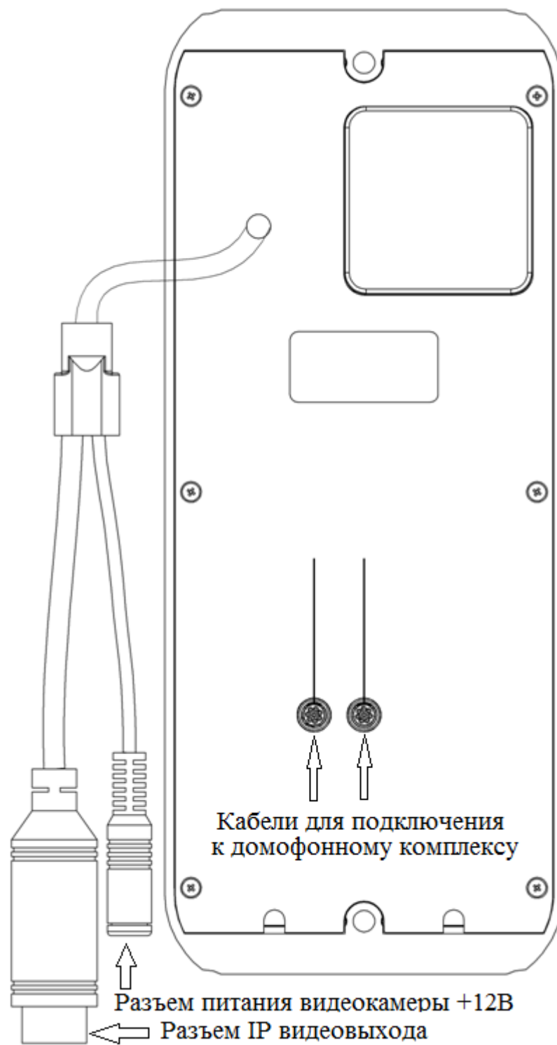
Рис.4 Внешний вид БВ DP5000.B2-KEDC43 IP307 и DP5000.B2-KEDC44 IP307 со стороны задней крышки
