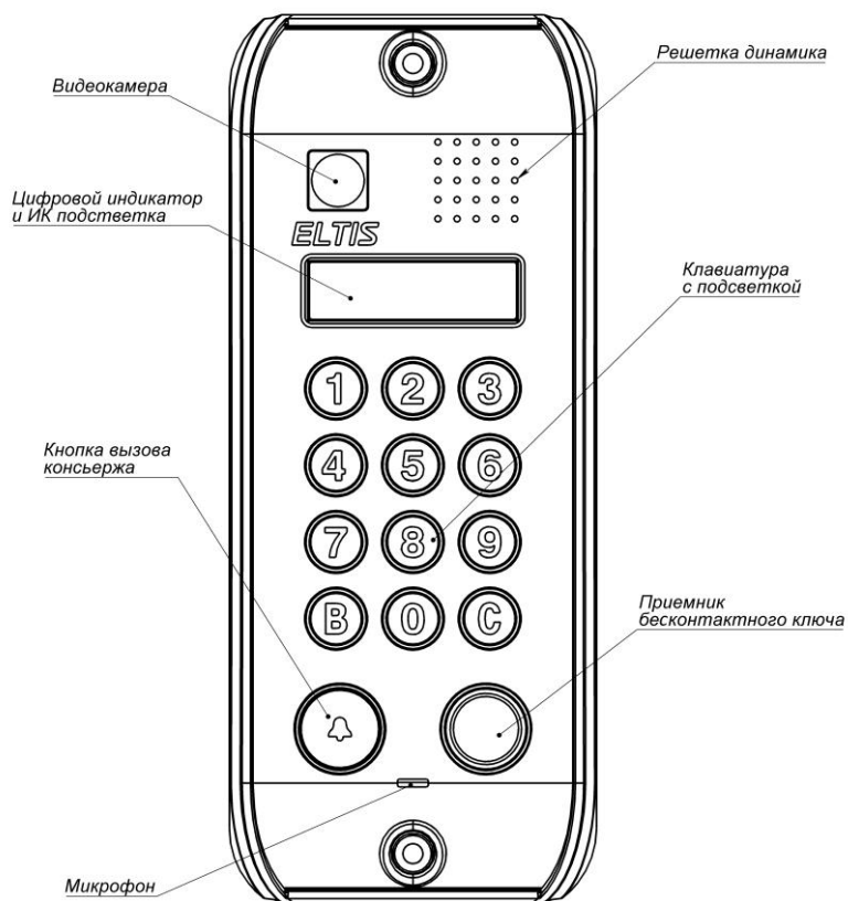
Рис.2.1 Внешний вид со стороны лицевой панели
