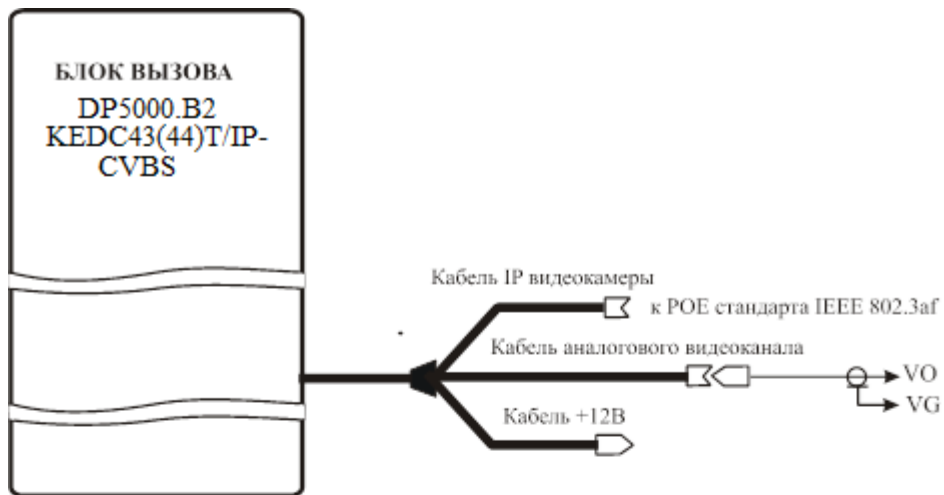
Схема подключения видео с помощью POE стандарта IEEE 802.3af
